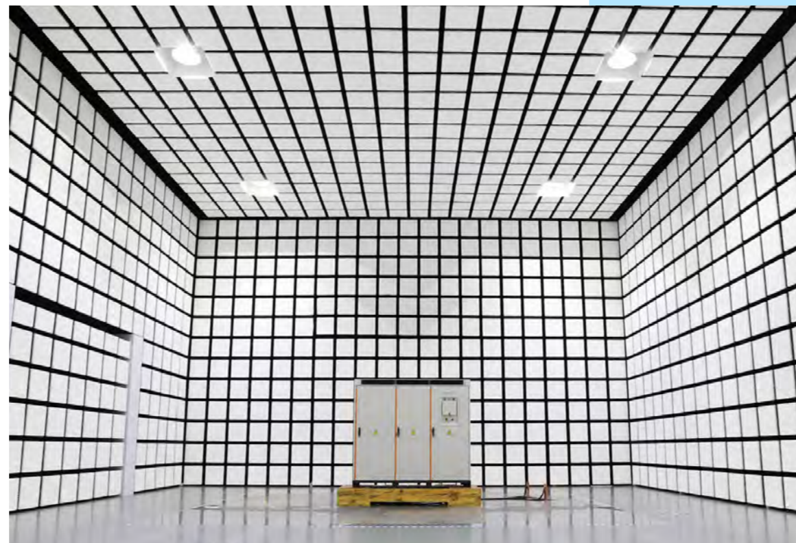
Quartier generale Sungrow a Hefei, Cina: La più grande camera EMC del settore solare
